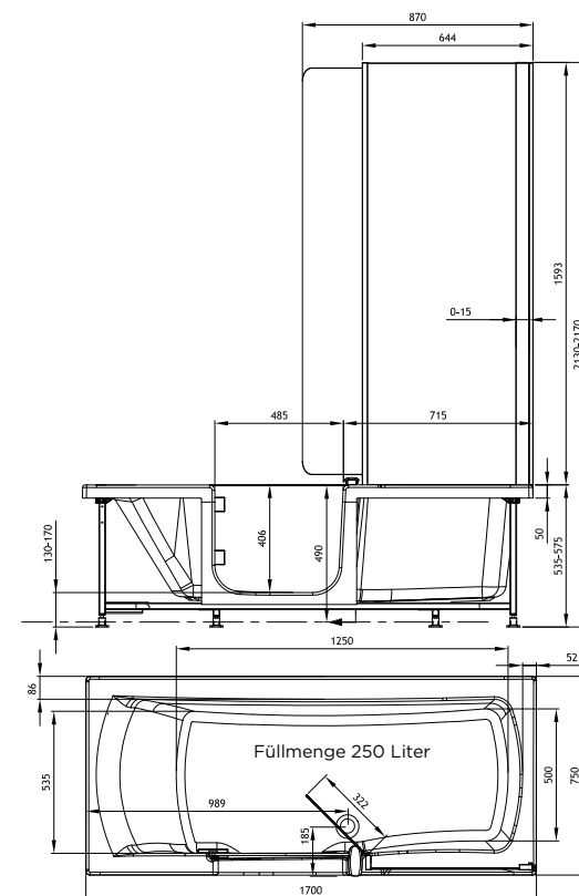
Version 170 x 75 cm, Kopfteil links
