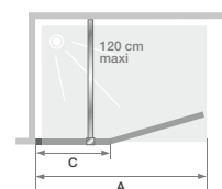
Größen \geq 110 cm Installation wahlweise links/rechts
