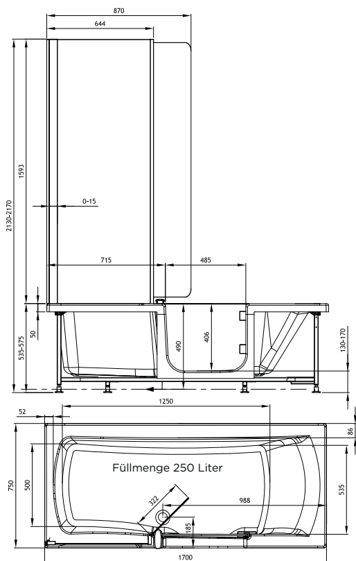
Version 170 x 75 cm, Kopfteil rechts
