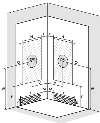
Abmessungen in cm
