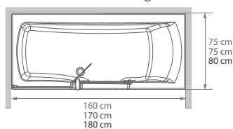
Nischenausführung mit festen Abmessungen
