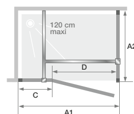
Größen \geq 110 cm Installation wahlweise links/rechts
