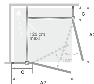
Installation wahlweise links/rechts
