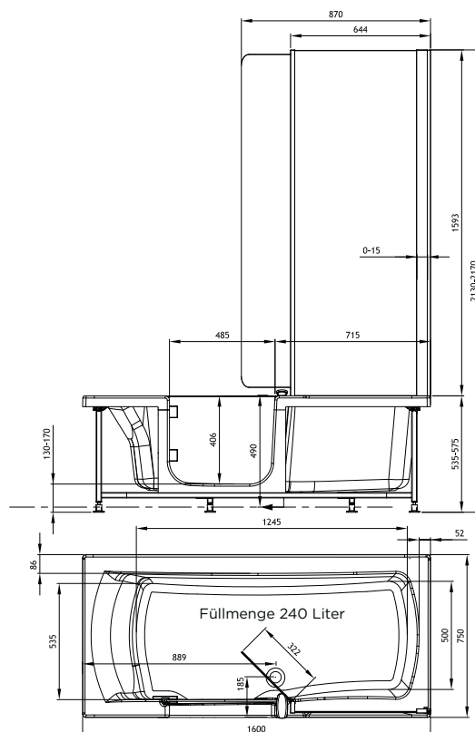
Version 160 x 75 cm, Kopfteil links
