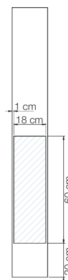
Wasseranschlussbereich
