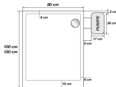
Pumpe rechts
