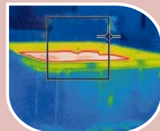
Mit Extra-Wärmedämmung: Die Wärme bleibt im Whirlpool
