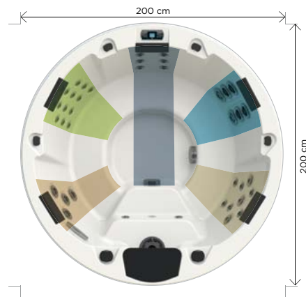
Höhe 78 cm / Fassungsvermögen: 700 l
